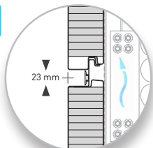
LONGITUDINAL JOINT
